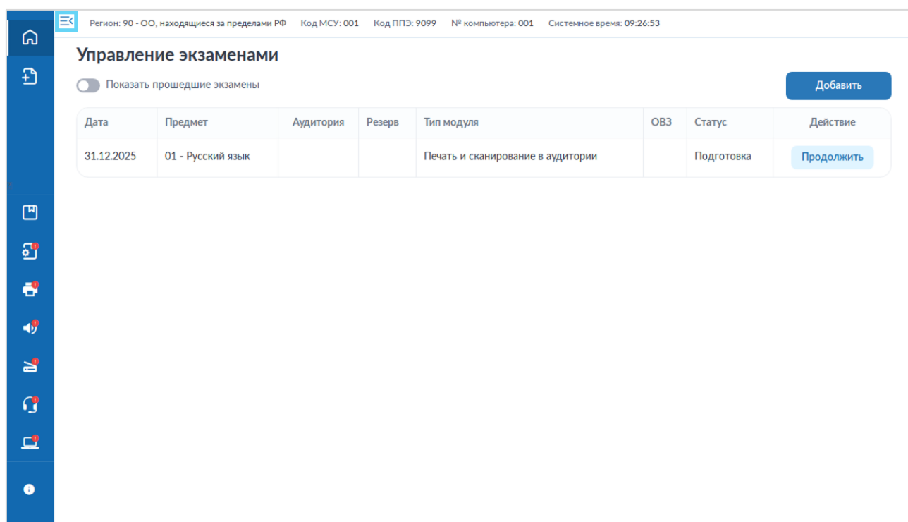
Рис. 3.8. Меню свернуто
